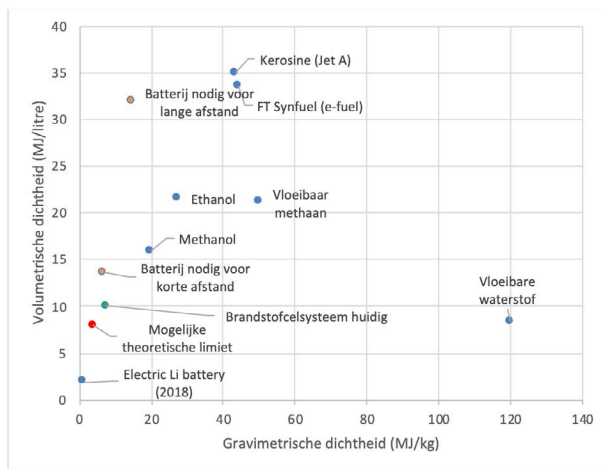
Figuur 4: Overzicht van de energiedichtheid met betrekking tot gewicht en volume voor kerosine, alternatieve brandstoffen en batterijen, brandstofcelsysteem huidige technologie op diverse studies.
