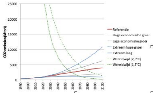
Figuur 1: Ontwikkeling van de lange-termijn wereldwijde CO 2 emissies van luchtvaart en de in de twee Parijse doelscenario's afgesproken emissies voor alle sectoren samen. Bron: (Peeters, 2017).
