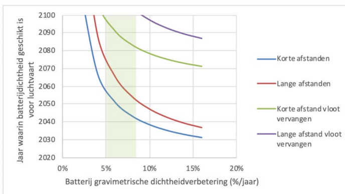
Figuur 5: implementatie van elektrisch vliegen als functie van het tempo waarin de dichtheid van batterijen groter wordt. Historische tempo varieerde tussen 5% en 8% per jaar (de groene band).
